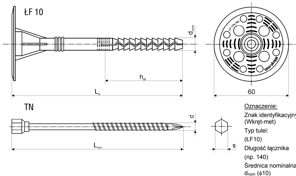
Tablica 2: Oznaczenia i wymiary [mm] łączników WKRET-MET-ŁFMΦ10
