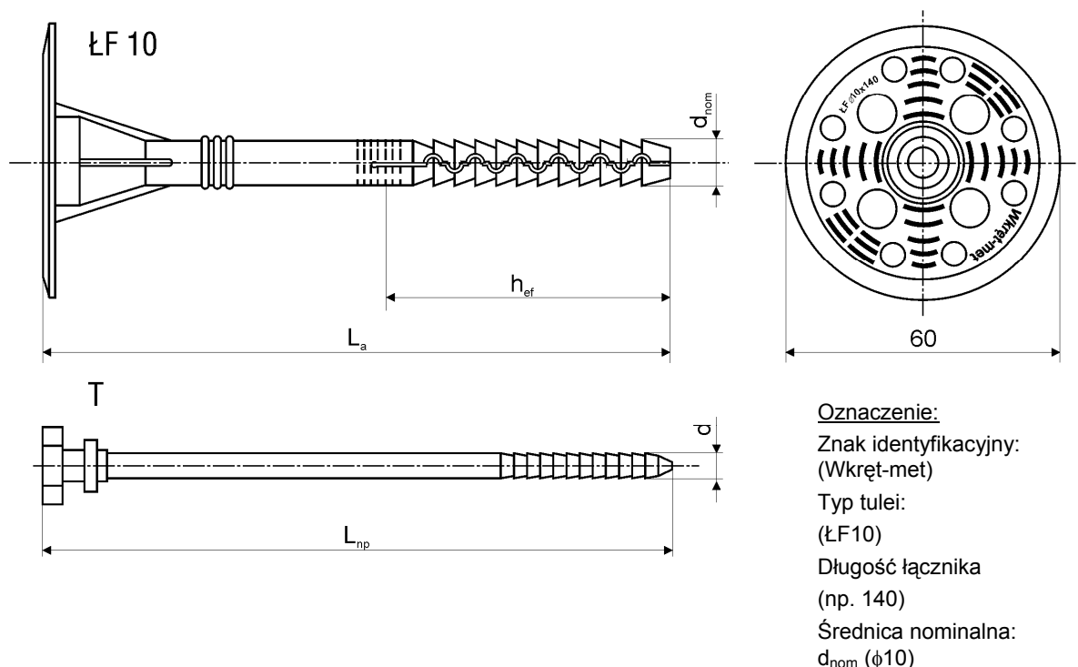
Tablica 1: Oznaczenia i wymiary [mm] łączników WKREĆ-MET-ŁFN \phi 10
